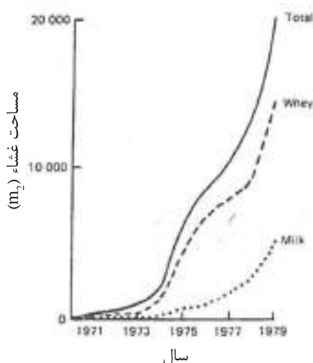
شکل ۵: مساحت غشای اولترافیلتراسیون در صنایع لبنیات-رشد در مدت ۱۰ سال ۱۹۷۰-۱۹۸۰؛ (داده‌ها از پنج کارخانه-بکور، دی.دی.اس، پی.سی.آی، رون-پولنک و رومیکون بدست آمده است).
